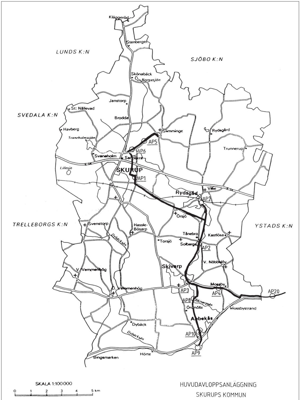
Figur 1. Översiktlig kartskiss över huvudavloppsledningen från Skurup till Ystad som den blev utförd. Källa: Skurups kommuns tekniska nämnd.
