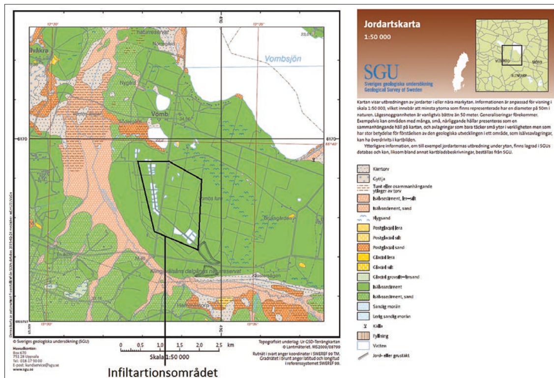
Fig. 3. Jordartskarta över sydvästra Vombsjöområdet (©Sveriges geologiska undersökning, 2015).
